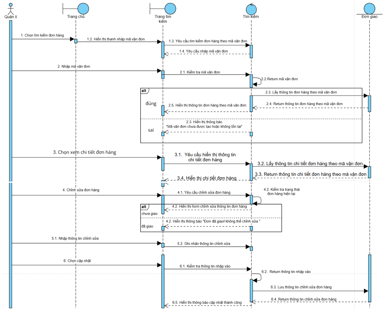
Hình 3.6.2.2. Sequence Diagram chức năng chỉnh sửa và cập nhật đơn giao
