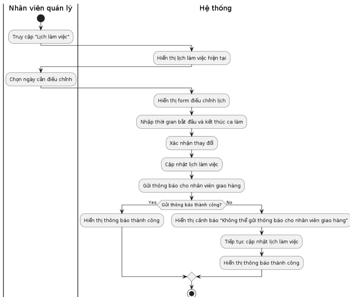
Hình 3.13.2.1. Activity Diagram chức năng điều chỉnh lịch làm việc
