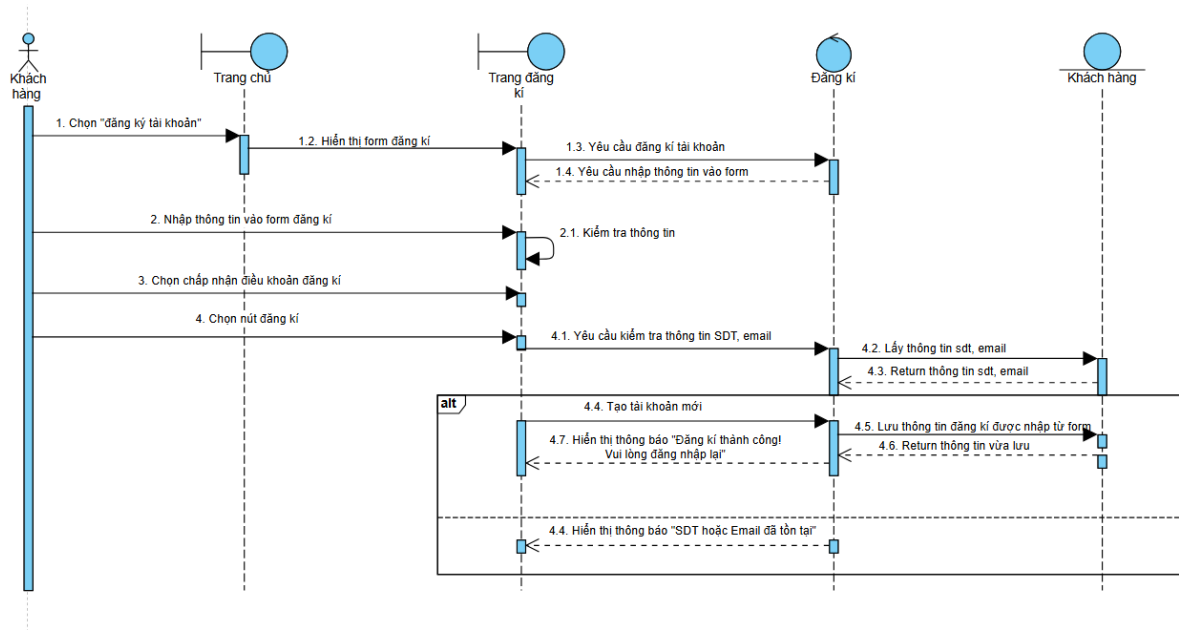
Hình 3.1.2.2. Sequence chức năng đăng kí
