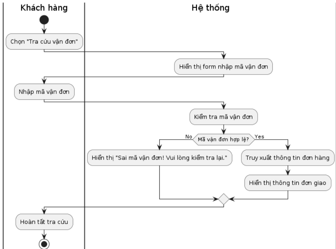
Hình 3.4.2.1 Activity Diagram chức năng theo dõi vận đơn
