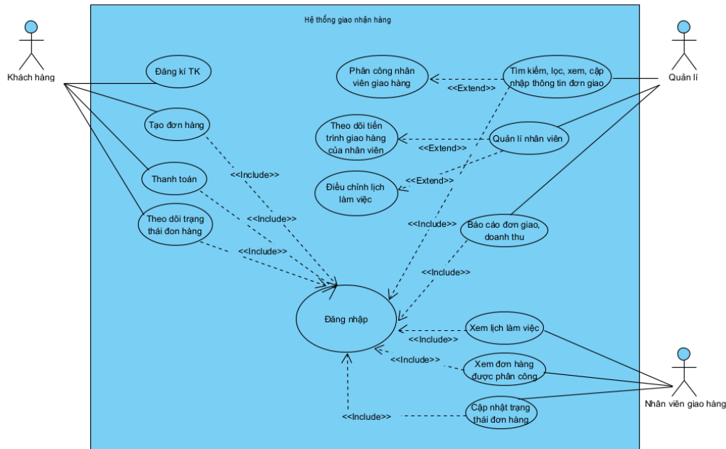
Hình 3.1.1. Sơ đồ use case
