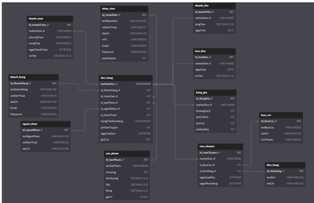
Hình 4.1 Cơ sở dữ liệu của hệ thống
