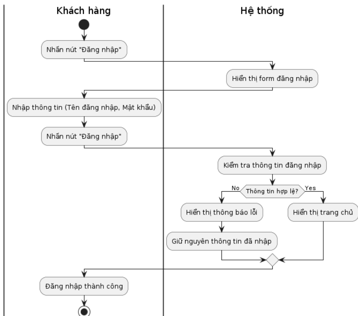
Hình 3.2.2.1. Activity Diagram chức năng đăng nhập
