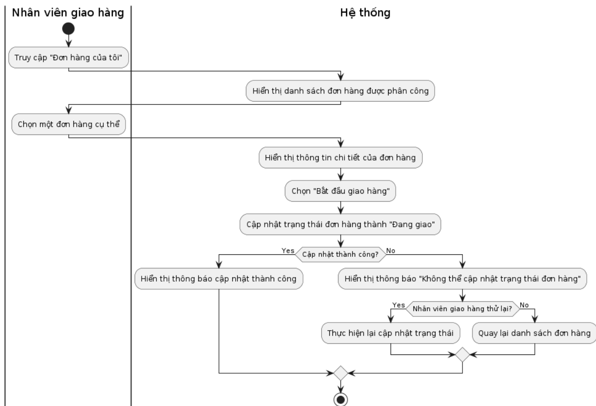
Hình 3.11.2.1. Activity Diagram chức năng xem đơn hàng được phân công
