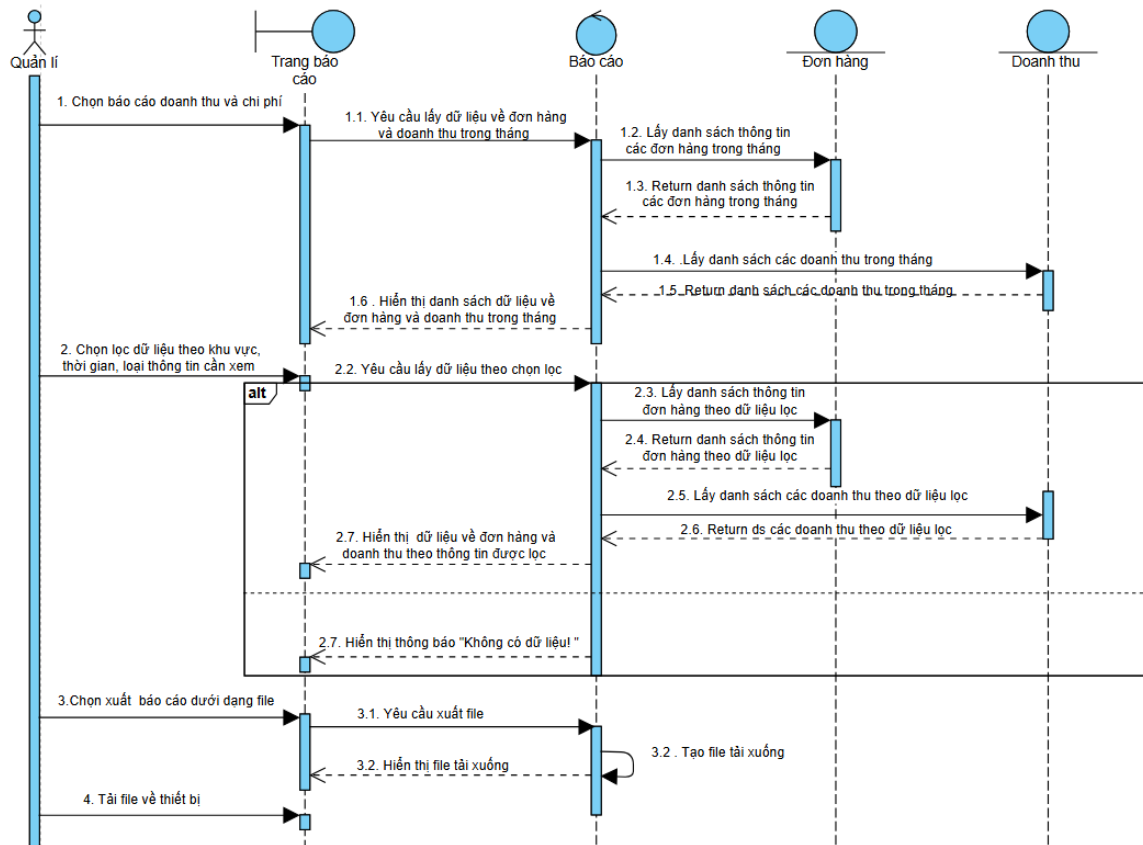
Hình 3.7.2.2. Sequence Diagram chức năng báo cáo đơn hàng và doanh thu
