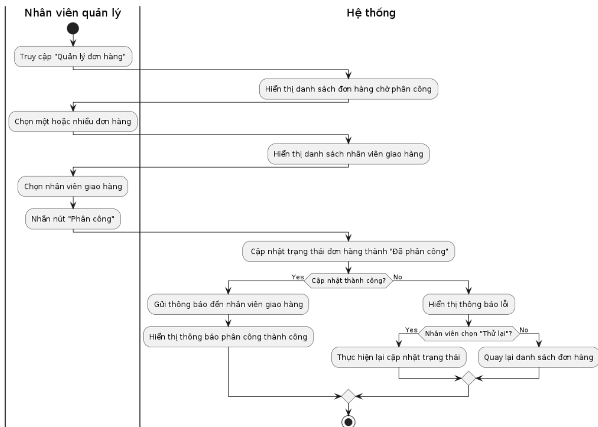
Hình 3.9.2.1. Activity Diagram chức năng phân công nhân viên giao hàng
