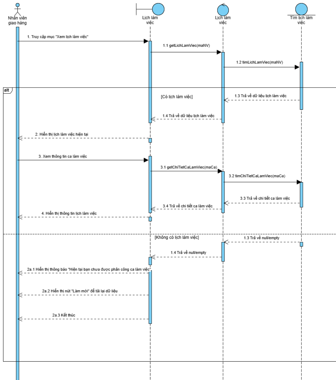
Hình 3.14.2.2. Sequence Diagram chức năng xem lịch làm việc
