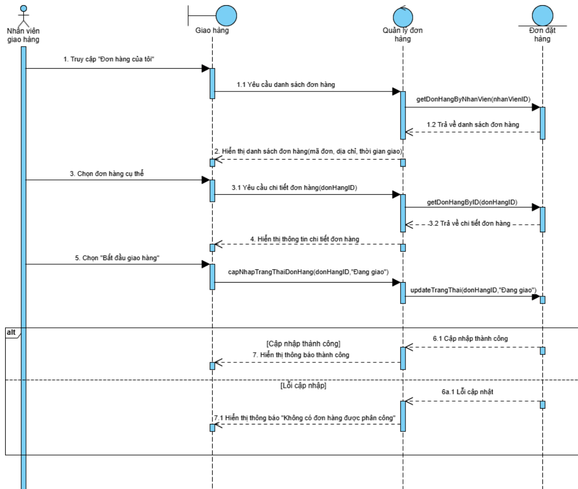
Hình 3.11.2.2. Sequence Diagram chức năng xem đơn hàng được phân công
