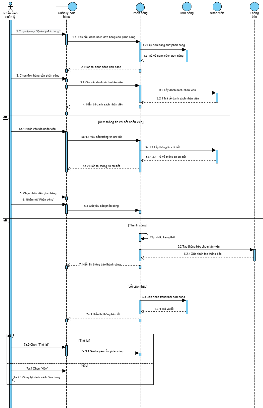
Hình 3.9.2.2. Sequence Diagram chức năng phân công nhân viên giao hàng
