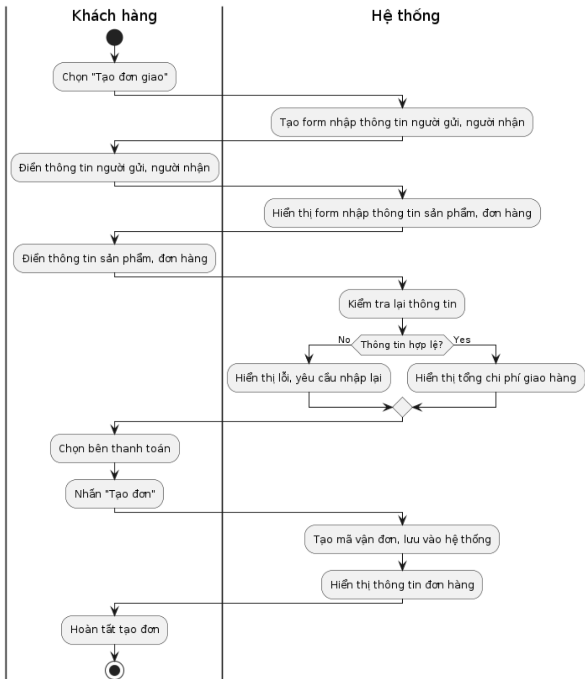
Hình 3.3.2.1. Activity Diagram chức năng tạo đơn giao
