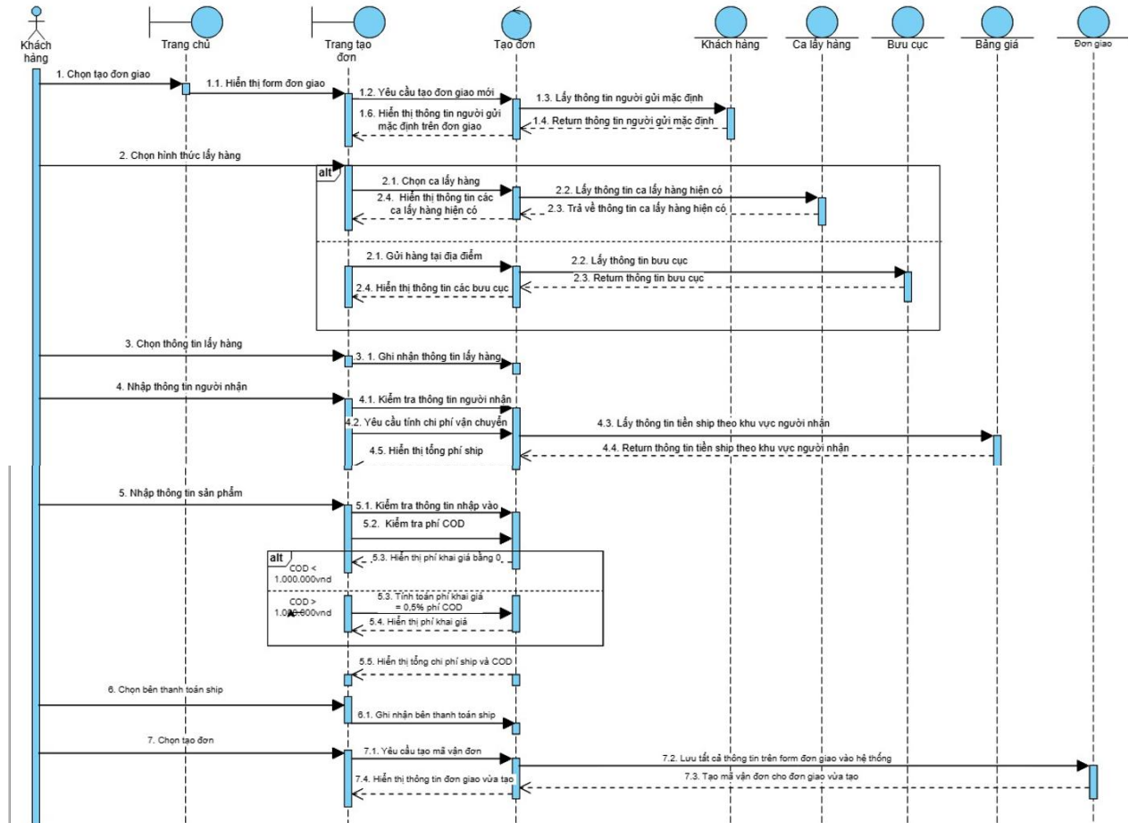
Hình 3.3.2.2. Sequence Diagram chức năng tạo đơn giao
