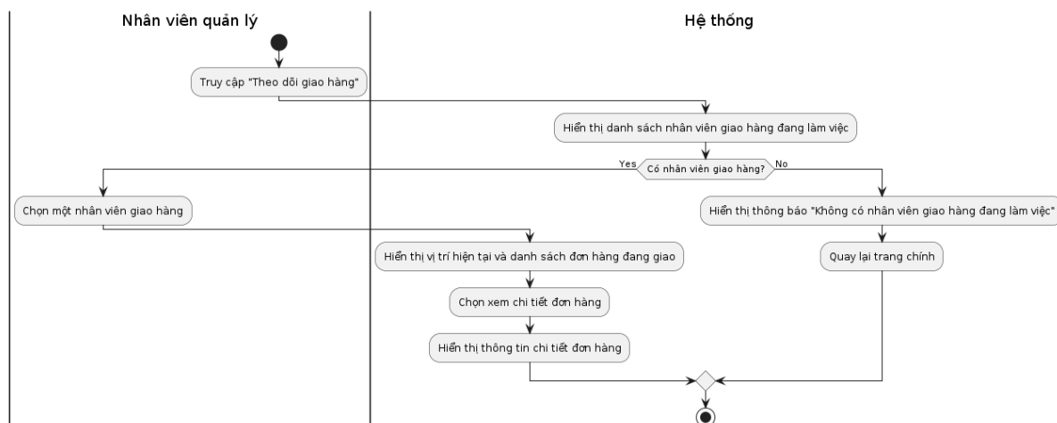
Hình 3.10.2.1. Activity Diagram chức năng theo dõi tiến trình giao hàng của nhân viên
