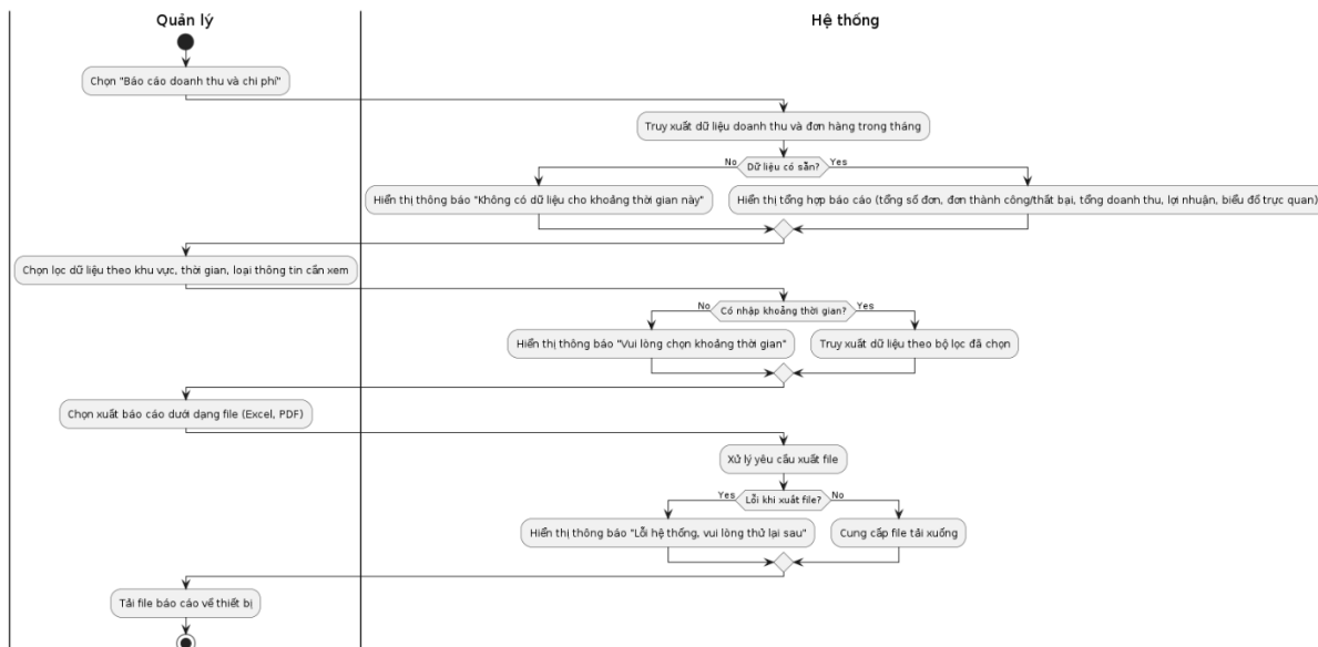
Hình 3.7.2.1. Activity Diagram chức năng báo cáo đơn hàng và doanh thu
