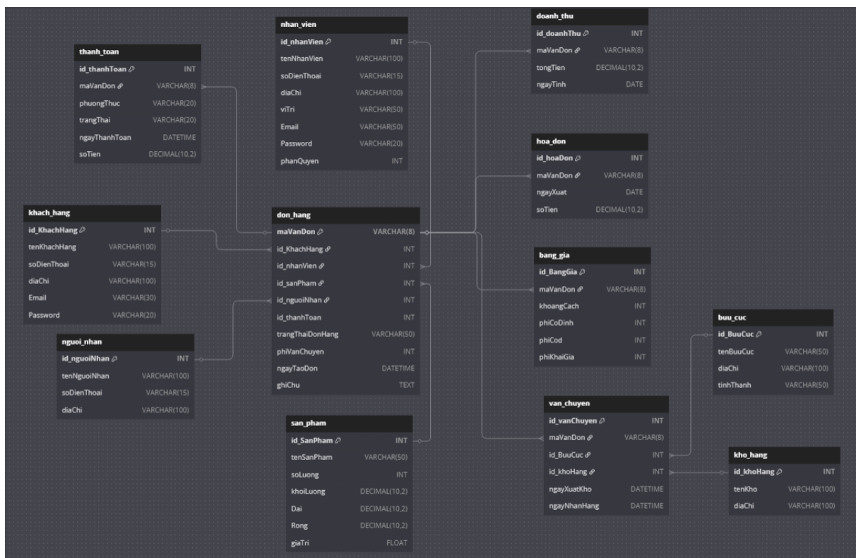
Hình 3.2.3. Class Diagram hệ thống
