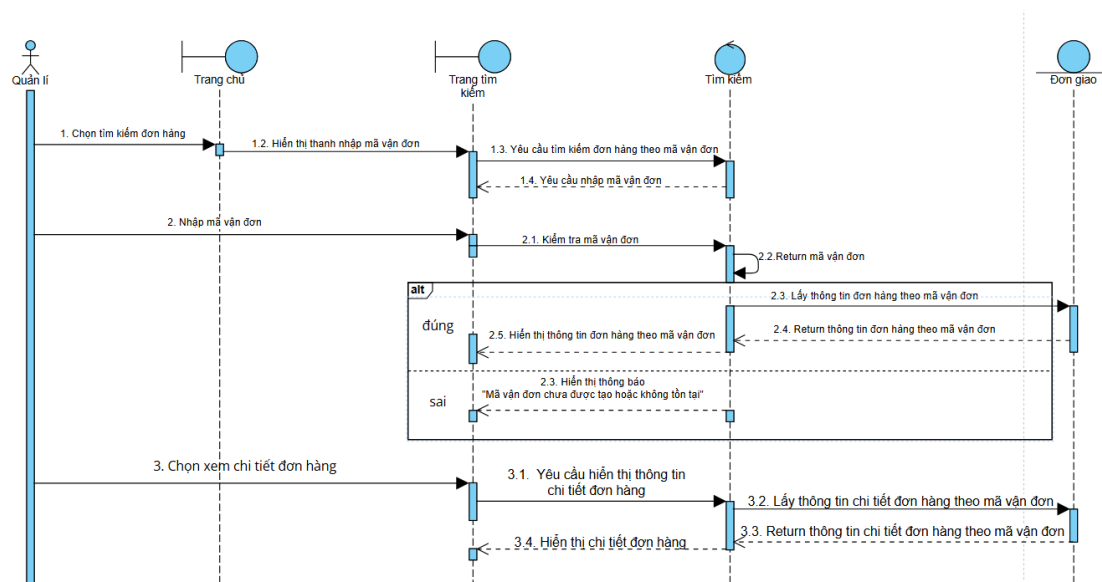
Hình 3.5.2.2. Sequence Diagram chức năng tìm kiếm và xem đơn giao
