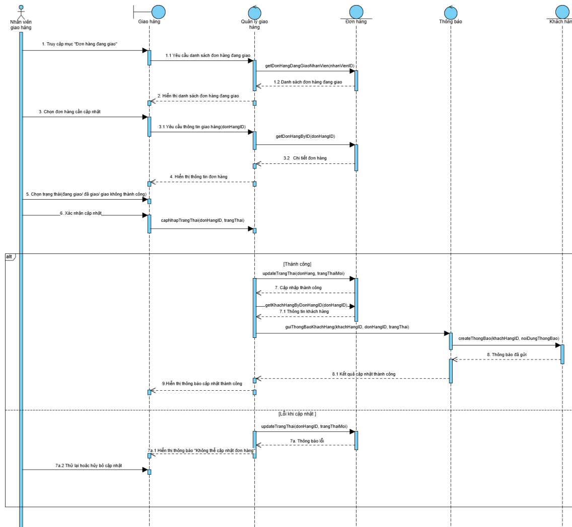
Hình 3.12.2.2. Sequence Diagram chức năng cập nhật trạng thái đơn hàng
