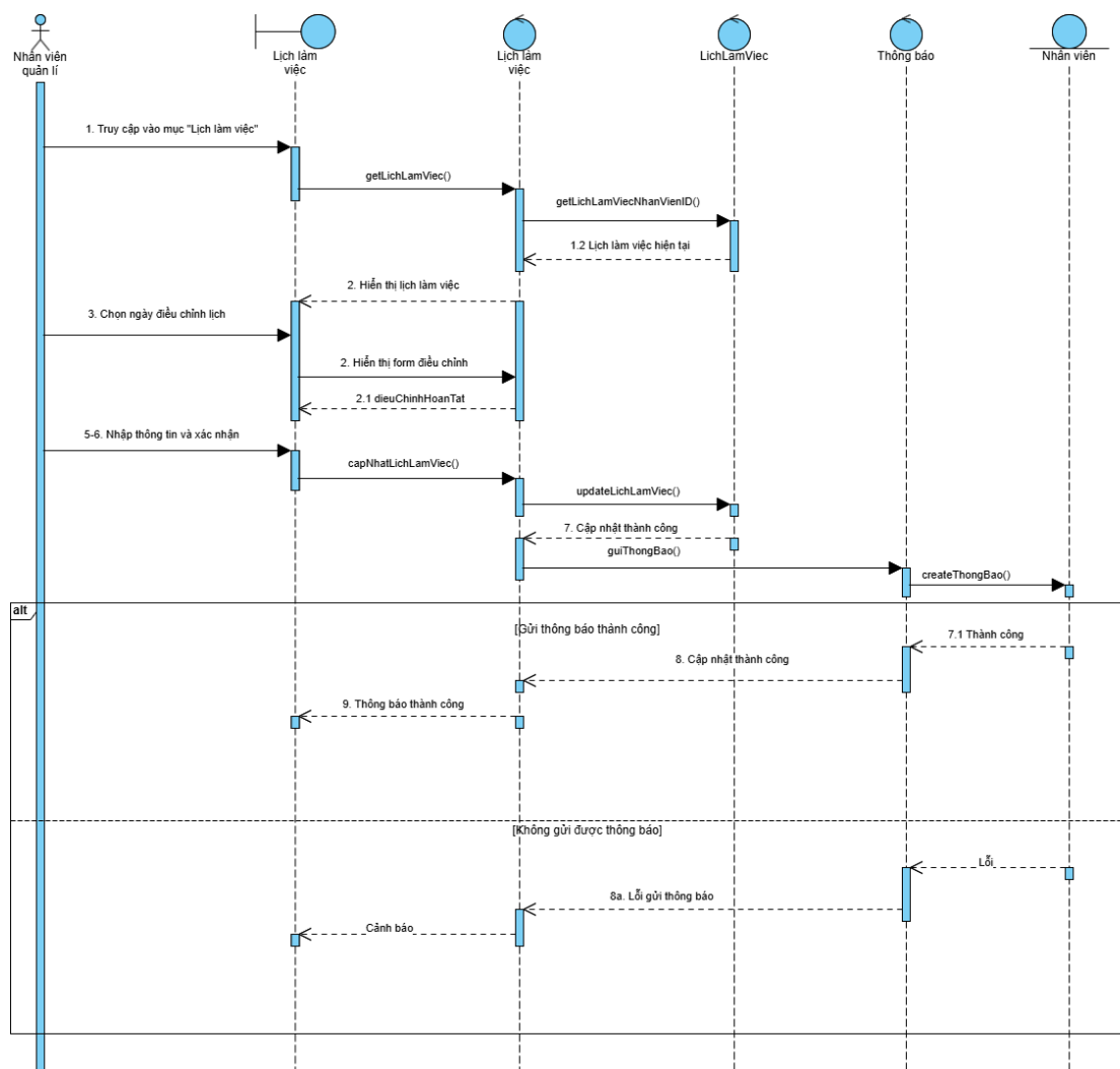
Hình 3.13.2.2. Sequence Diagram chức năng điều chỉnh lịch làm việc
