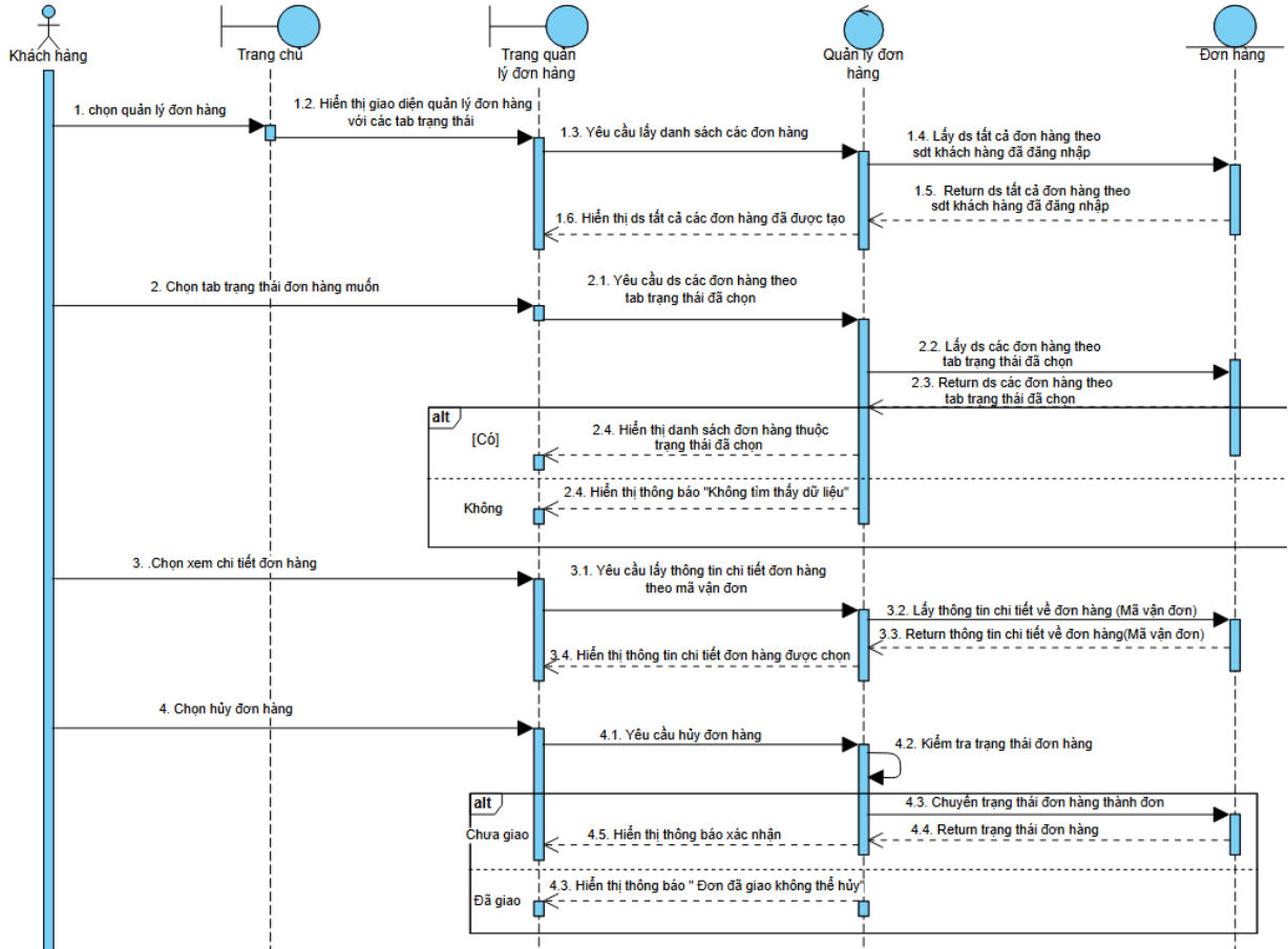
Hình 3.8.2.2. Sequence Diagram chức năng quản lý đơn hàng
