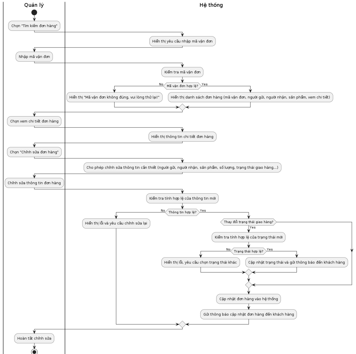
Hình 3.6.2.1. Activity Diagram chức năng chỉnh sửa và cập nhật đơn giao
