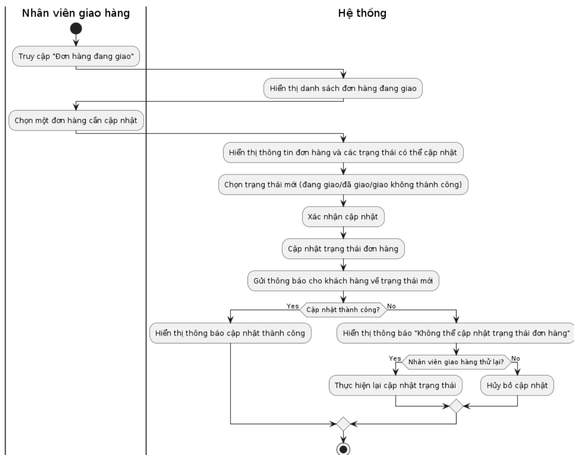
Hình 3.12.2.1. Activity Diagram chức năng cập nhật trạng thái đơn hàng
