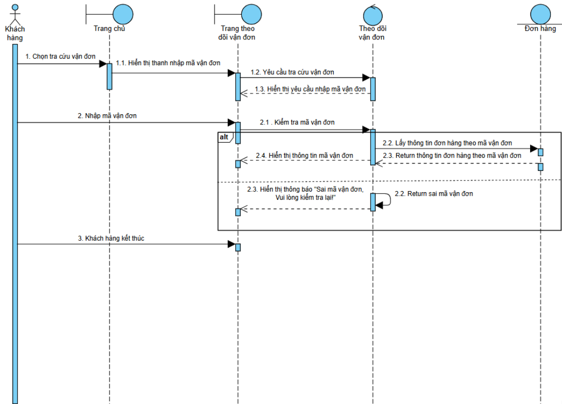
Hình 3.4.2.2. Sequence Diagram chức năng theo dõi vận đơn
