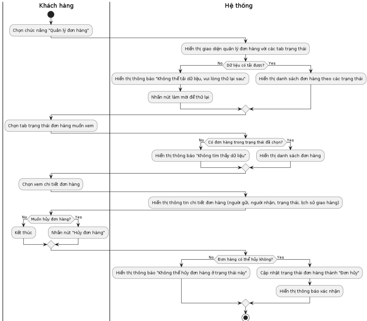
Hình 3.8.2.1. Activity Diagram chức năng quản lý đơn hàng
