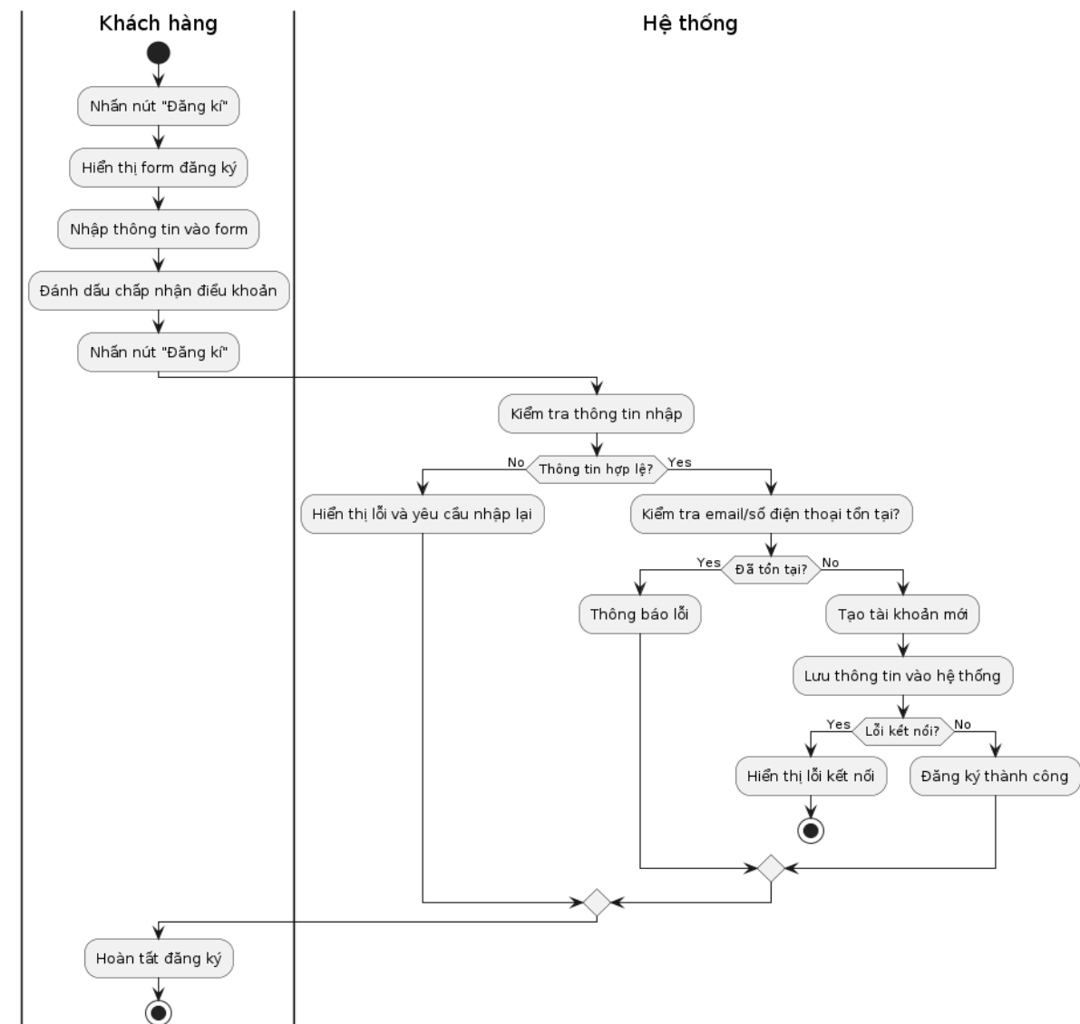
Hình 3.1.2.1. Activity Diagram chức năng đăng kí
