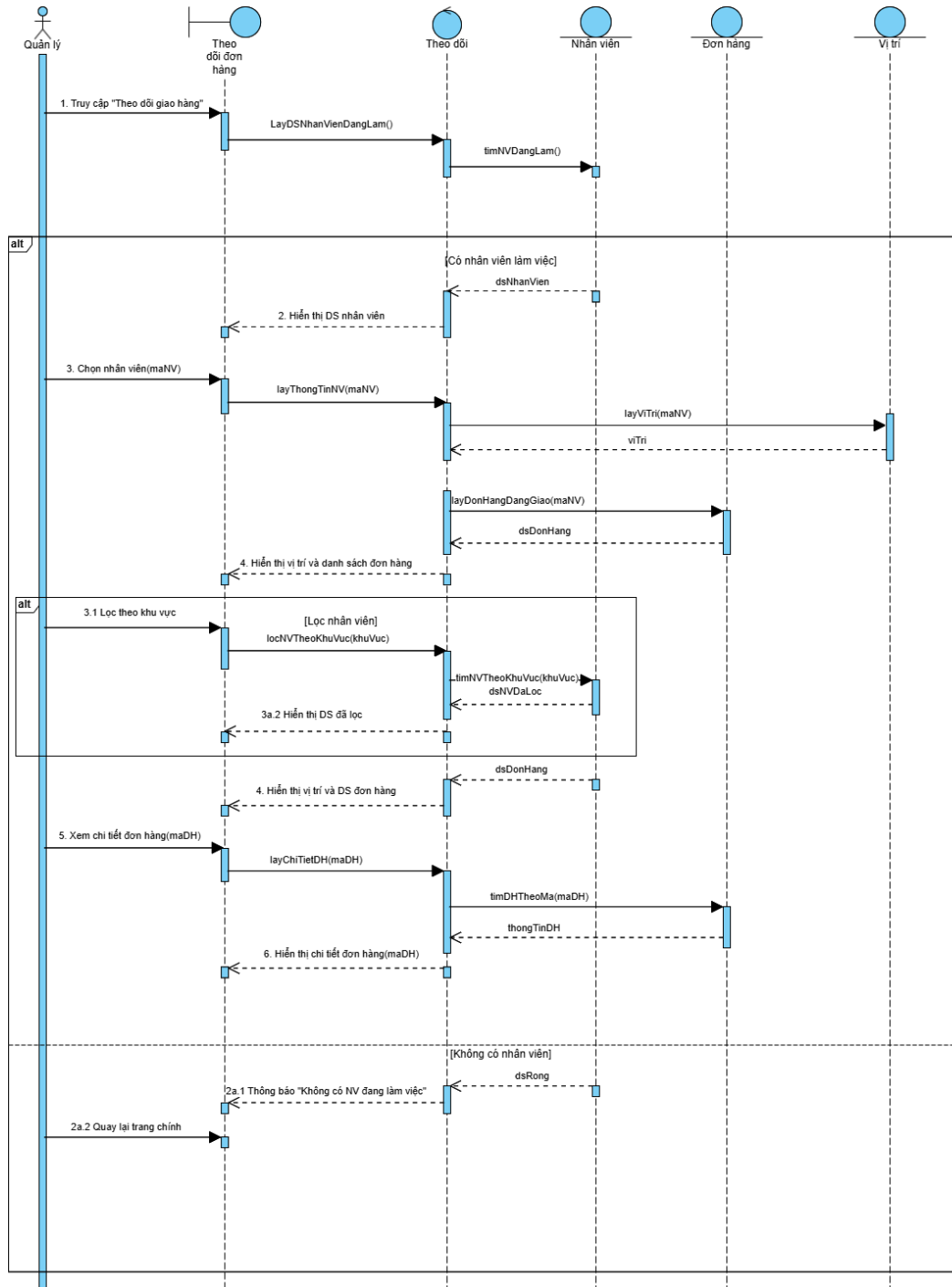
Hình 3.10.2.2. Sequence Diagram chức năng theo dõi tiến trình giao hàng của nhân viên
