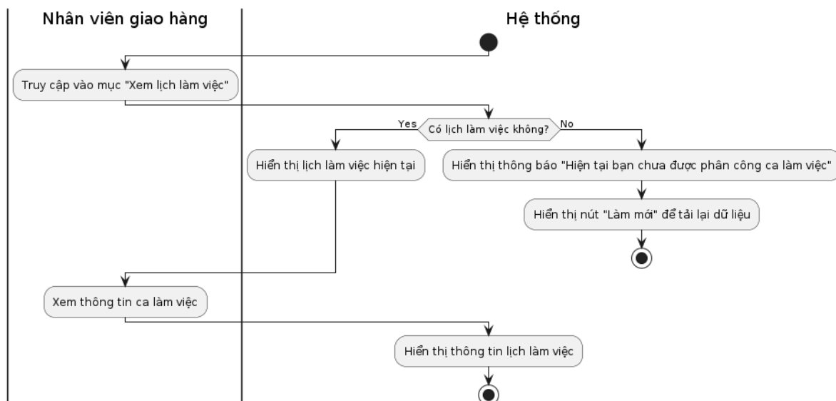
Hình 3.14.2.1. Activity Diagram chức năng xem lịch làm việc
