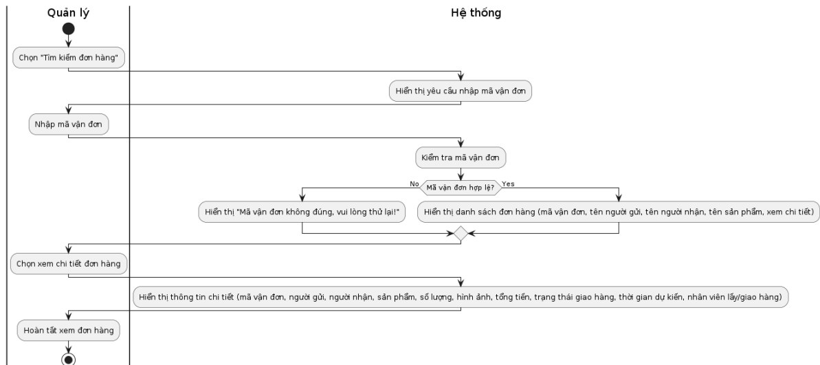
Hình 3.5.2.1. Activity Diagram chức năng tìm kiếm và xem đơn giao
