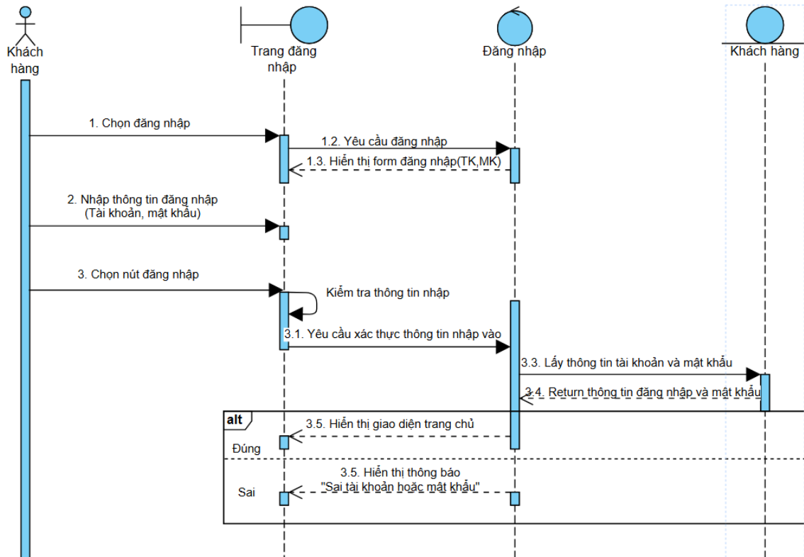
Hình 3.2.2.2. Sequence Diagram chức năng đăng nhập
